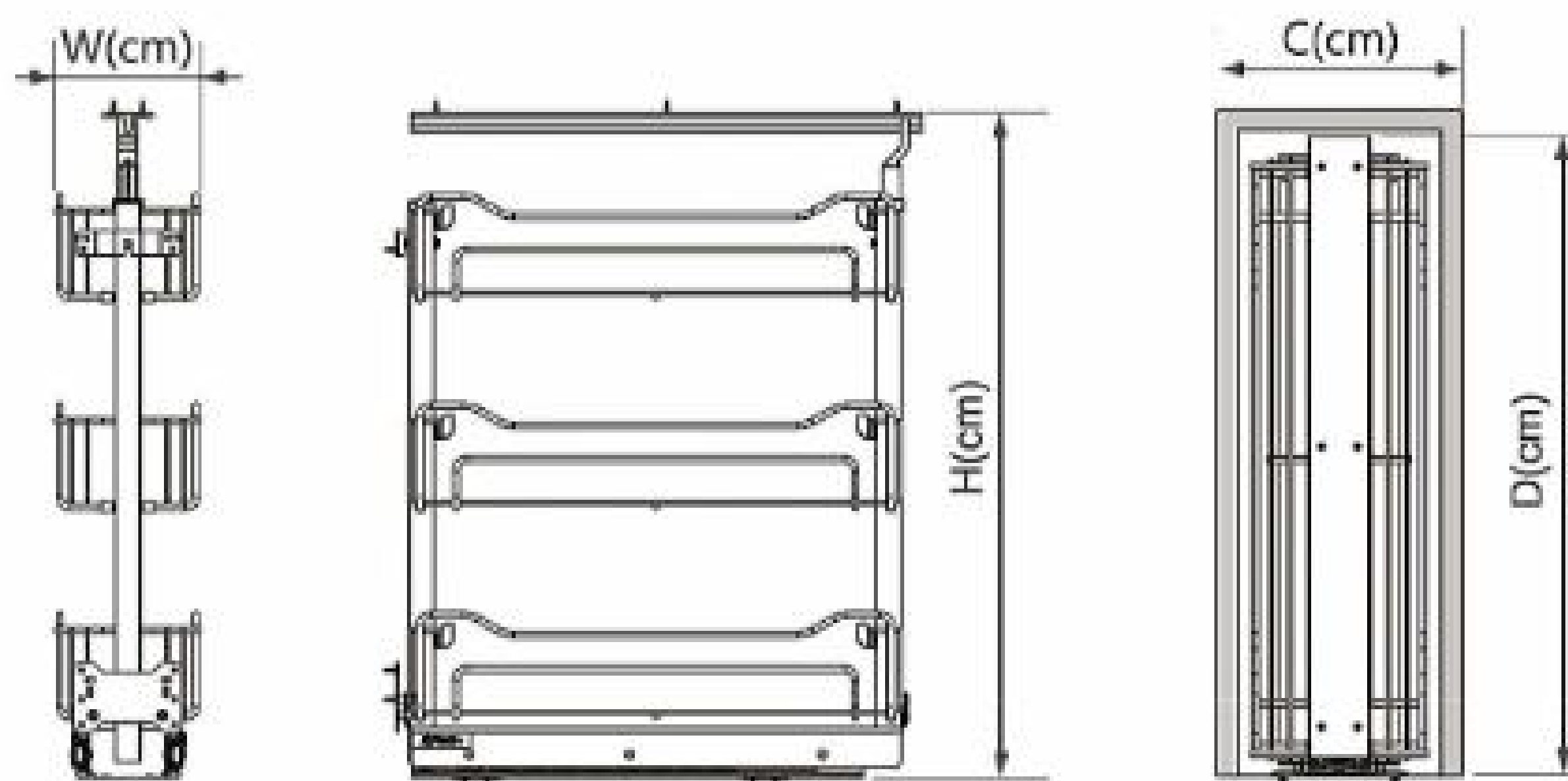
Stabilization mechanism مکانیزم لرزه گیر
